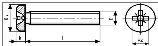
DIN 7985
