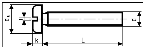
DIN 85
