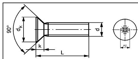
DIN 965
